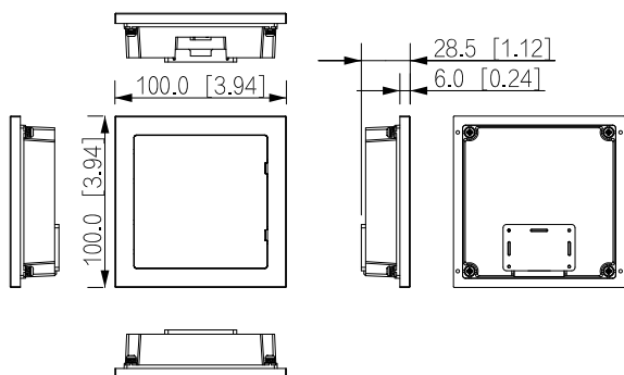
DHI-VTO4202F-MI
