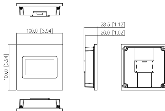
DHI-VTO4202F-MS
