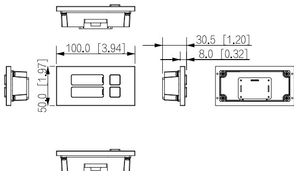
DHI-VTO4202F-MB2
