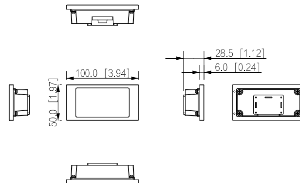
DHI-VTO4202F-MR.DHI-VTO4202F-MR1
