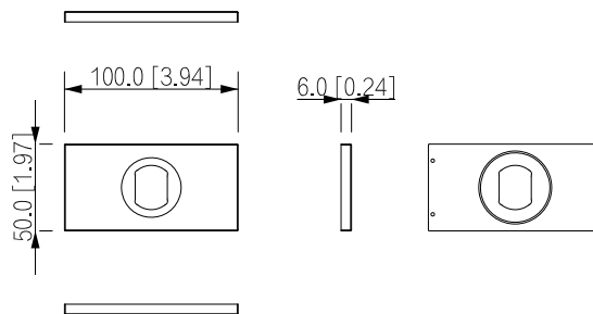
DHI-VTO4202F-MV
