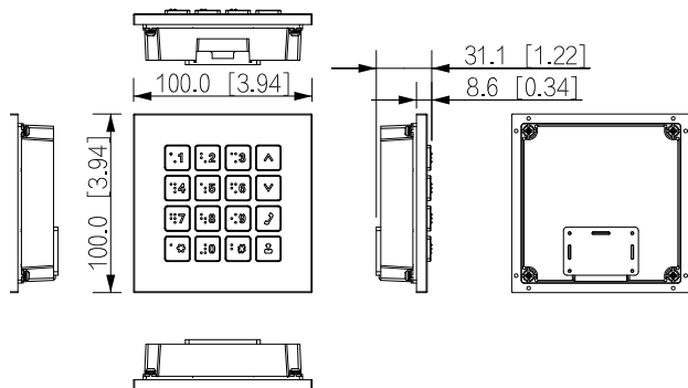
DHI-VTO4202FB-MK
