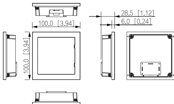
DHI-VTO4202FB-MI
