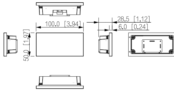
DHI-VTO4202FB-MN
