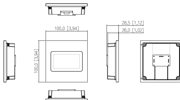
DHI-VTO4202FB-MS
