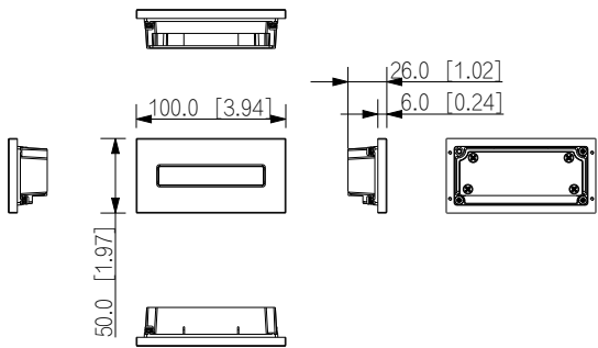
DHI-VTO4202FB-MDB2
