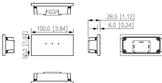
DHI-VTO4202FB-ML
