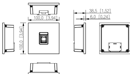
DHI-VTO4202FB-MF
